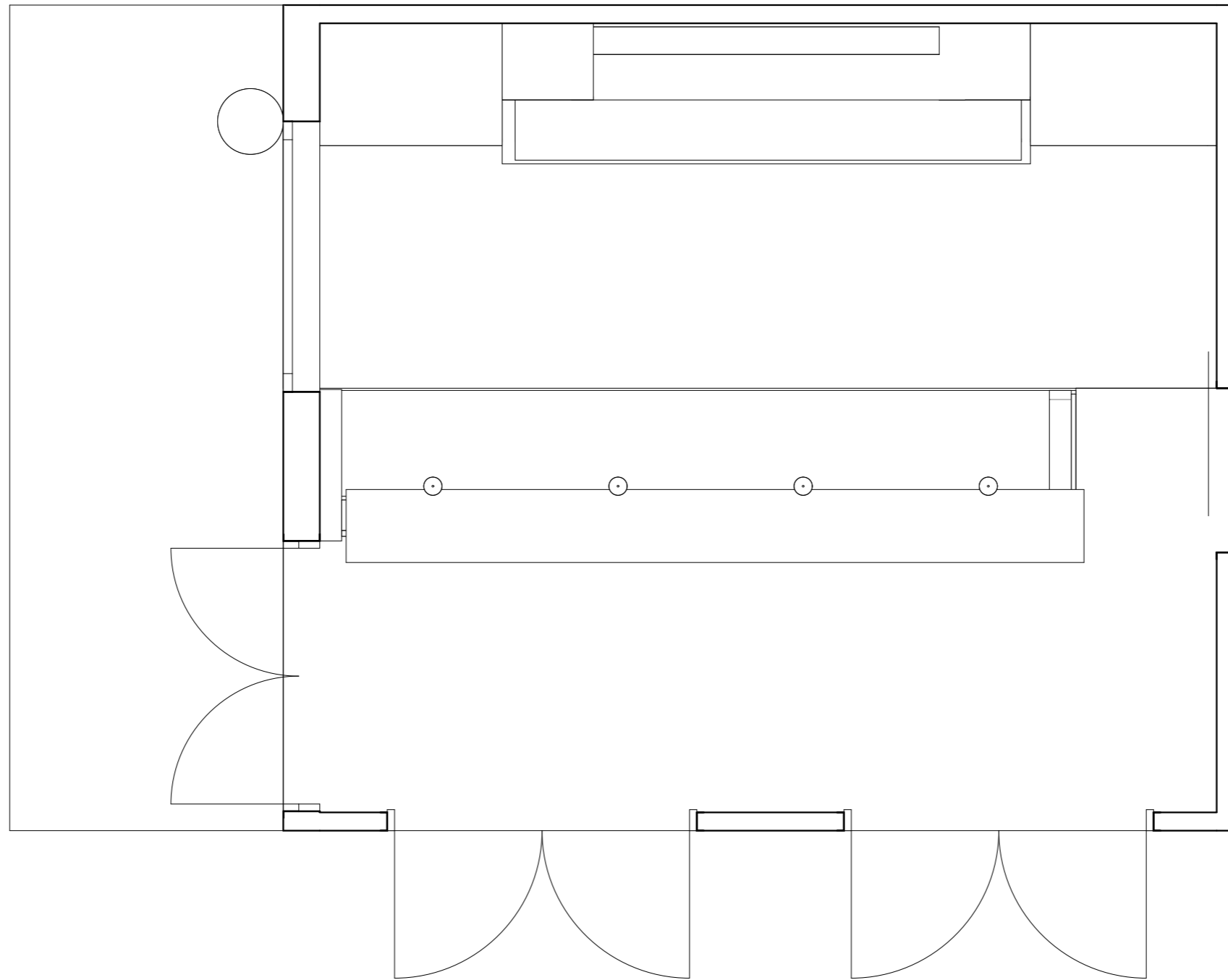
PLAN, 1:30
